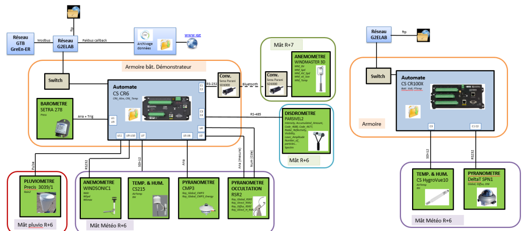
Fig.4 : système de mesure
