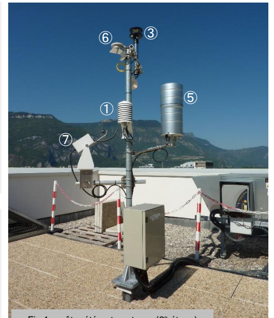
Fig.1 : mât météo et capteurs (6 e étage)
