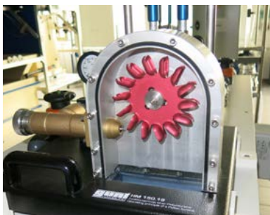
Modèle réduit de roue Pelton
